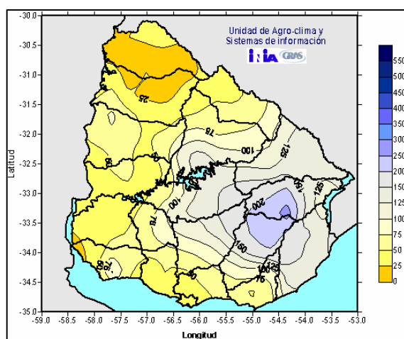
Precipitaciones en agosto de 2006
