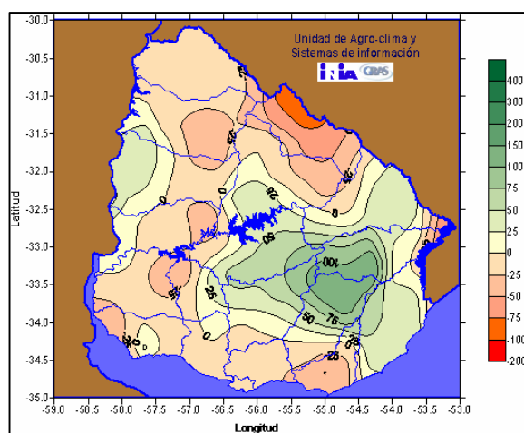
Anomalías de precipitación para agosto de 2006
