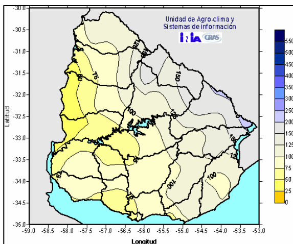
Precipitaciones en agosto de 2007
