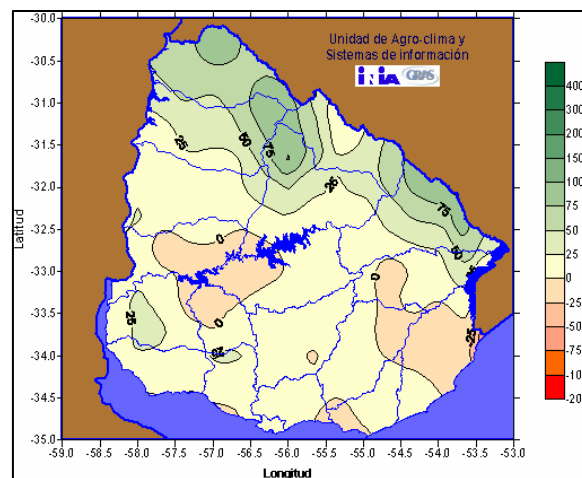
Anomalías de precipitación para agosto de 2007
