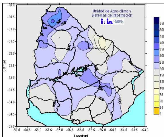
Precipitaciones en octubre de 2007
