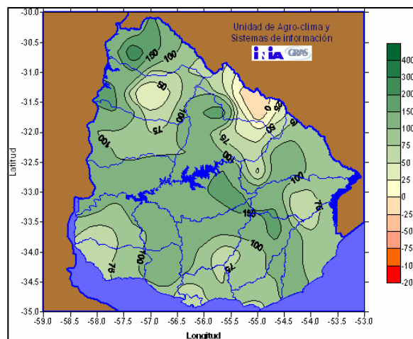
Anomalías de precipitación para octubre de 2007
