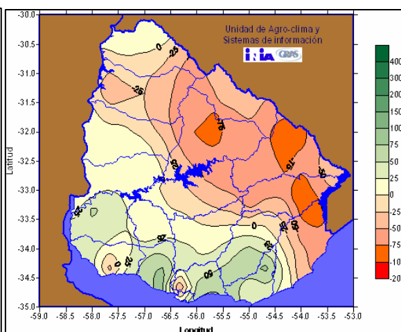
Anomalías de precipitación para setiembre de 2007
