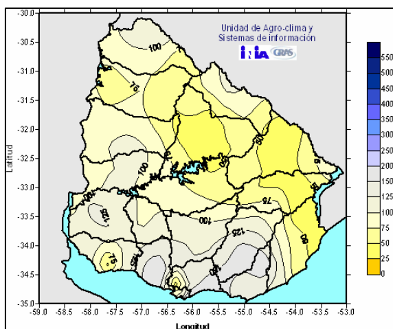
Precipitaciones en setiembre de 2007
