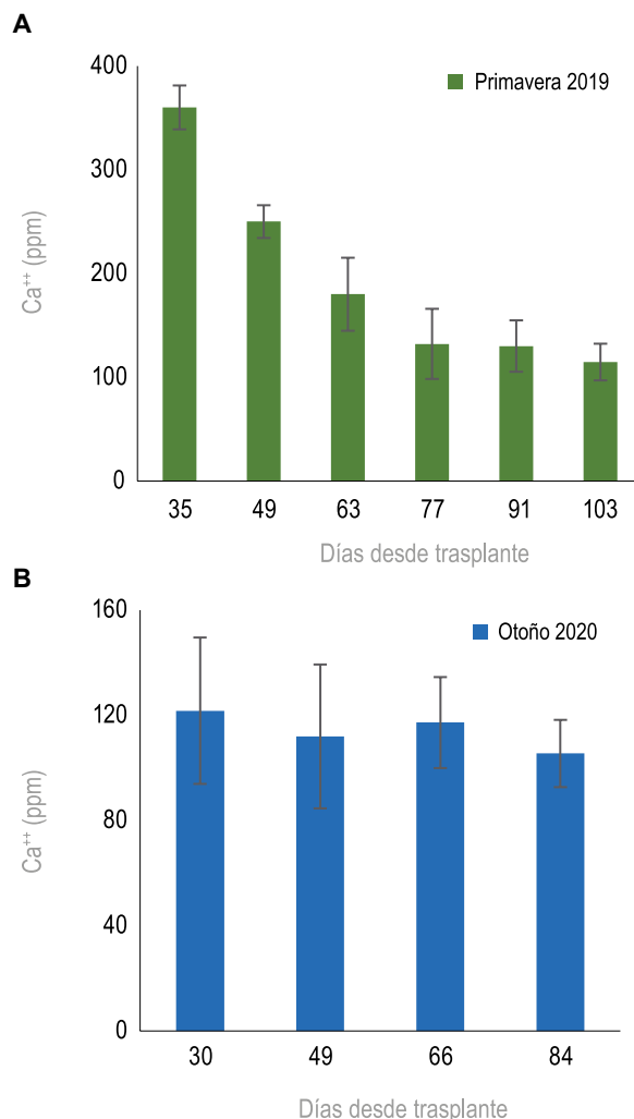
Figura 4 - Calcio en jugo de pecíolo a lo largo del ciclo del cultivo de tomate para Primavera 2019 (A) y Otoño 2020 (B).
